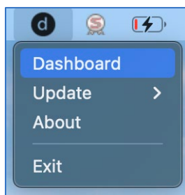
Слика 18
