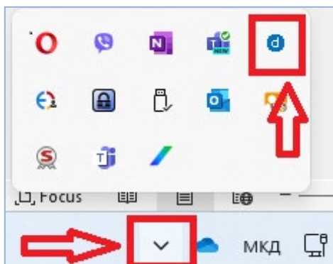
Слика 16
